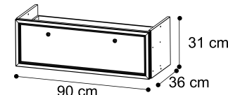
Elemento cestone L. 90 Large drawer unit L. 90
