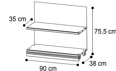
Fondo + Schiena + Ripiano Bottom + Back + Shelf
