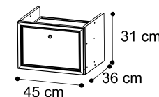
Elemento cestone L. 45 Large drawer unit L. 45
