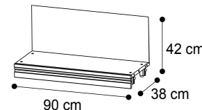
Fondo + Schiena Bottom + Back
