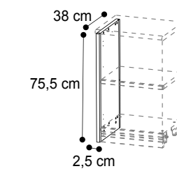
Fianco sinistro Left side
