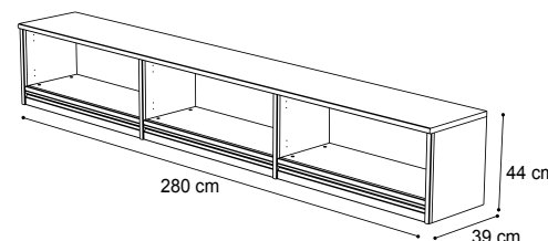
Base 3 moduli 3 module base
