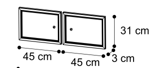
2 ante legno H. 31 2 woodens door H. 31
