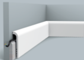
SX185 CASCADE 200 x 12 x 2,5 cm Duropolymer®
