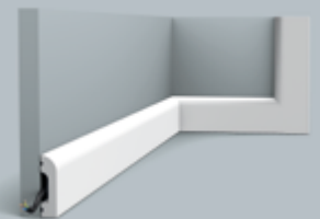
SX182 | SX182F CASCADE 200 x 5 x 1,3 cm Duropolymer®
