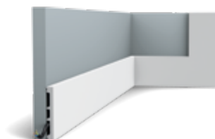
SX163 | SX163F SQUARE 200 x 10,2 x 1,3 cm Duropolymer®
