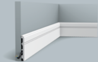
SX105 | SX105F 200 x 10,8 x 1,3 cm Duropolymer®
