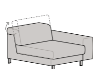
Poltrona Laterale Dx-Sx L 92 P 98 H 77/97 SLIM L 84 P 98 H 77/97
