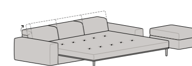
Componibile Panchetta Reversibile Letto L 256 P 230 H 77/97 SLIM L 240 P 230 H 77/97
