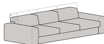
Divano L 256 P 98 H 77/97 SLIM L 240 P 98 H 77/97 1 o 2 RELAX lato bracciolo
