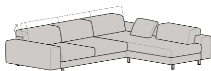
Componibile Penisola Reversibile L 256 P 195 H 77/97 SLIM L 240 P 195 H 77/97
