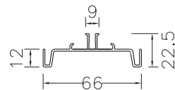
Sezione gola tipo "D" Type "D" finger rail section
