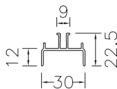
Sezione gola tipo "E" Type "E" finger rail section
