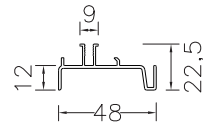
Sezione gola tipo "C" Type "C" finger rail section
