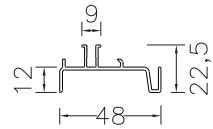
Sezione gola tipo "C" Type "C" finger rail section
