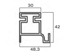
Sezione gola tipo "C" Type "C" finger rail section
