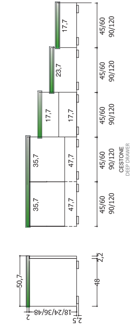
BASI LIVING CON PIEDINO H 2,5 ROOM UNITS WITH FEET H 2,5
