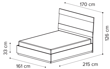
Letto KROMA 154x203 KROMA bed 154x203 Кровать KROMA 154x203
