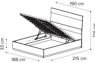
Letto KROMA c/contenitore e rete 180x200 KROMA bed with storage 180x200 Кровать KROMA с подъемным мех-мом 180x200
