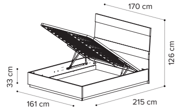
Letto KROMA c/contenitore e rete 154x203 KROMA bed with storage 154x203 Кровать KROMA с подъемным мех-мом 154x203
