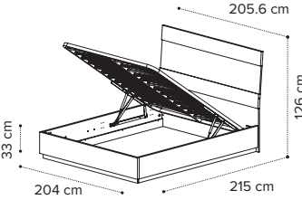
Letto KROMA c/contenitore e rete 195x203 KROMA bed with storage 195x203 Кровать KROMA с подъемным мех-мом 195x203
