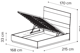
Letto KROMA c/contenitore e rete 160x200 KROMA bed with storage 160x200 Кровать KROMA с подъемным мех-мом 160x200
