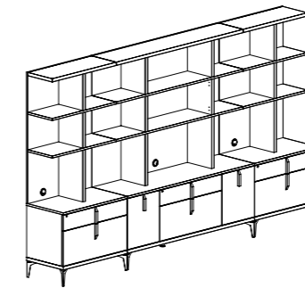
LIBRARY COMPOSITION 2 PJMM0801 inch W 142" D 20" H 84" cm L 360,8 P 52 H 212,2 Crts 10 kg 404 m 3 2,19
