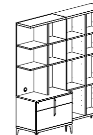
LIBRARY COMPOSITION 14 PJMM0813 inch W 75" D 20" H 84" cm L 190,6 P 52 H 212,2 Crts 6 kg 194 m 3 0,96
